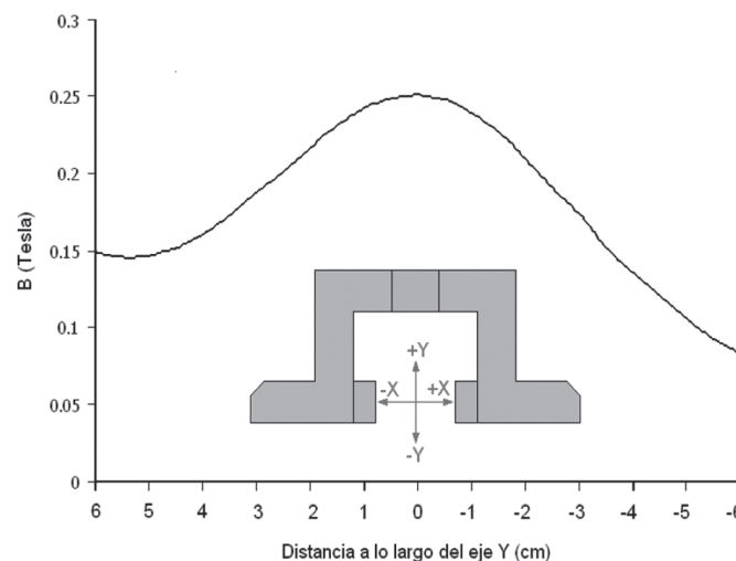
Fig. 4. Esquema del comportamiento del gradiente de campo a lo largo del eje y.
